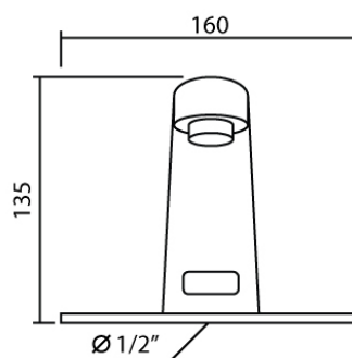
MODEL : MF-101 (mm.)
